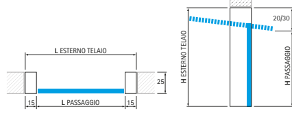
Posizione in luce
