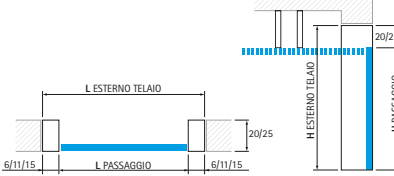
Posizione in luce
