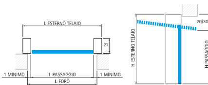
Posizione oltre luce
